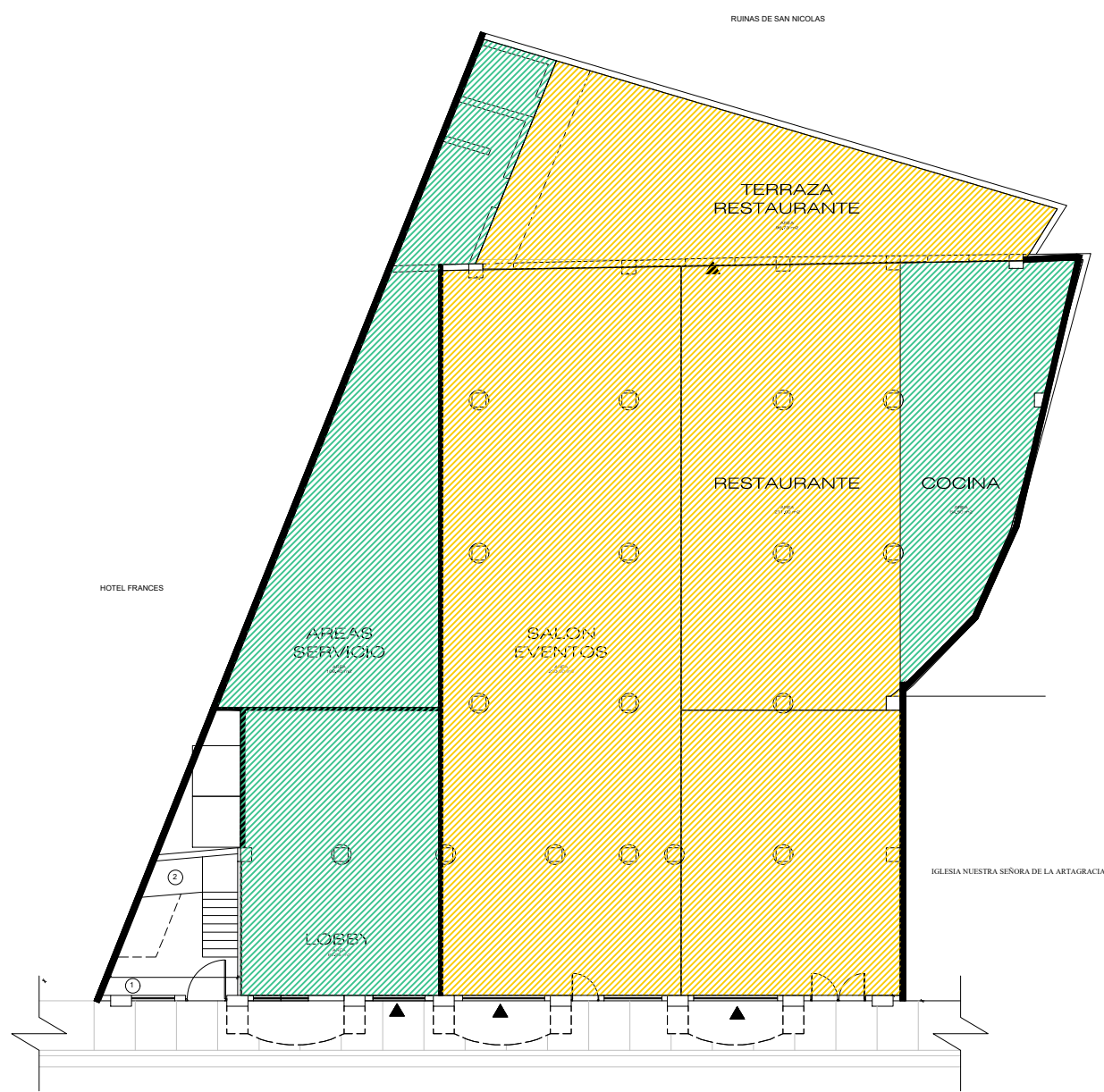
PLANTA PISO 1
