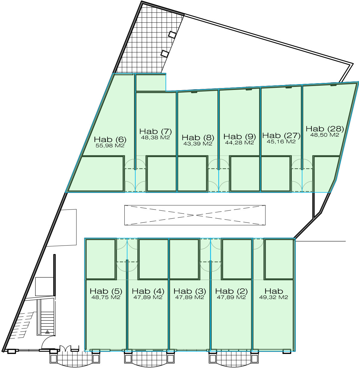
PLANTA PISO 2
