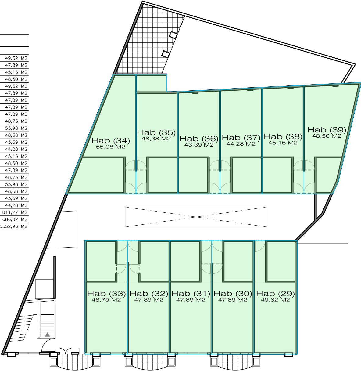
PLANTA PISO 3
