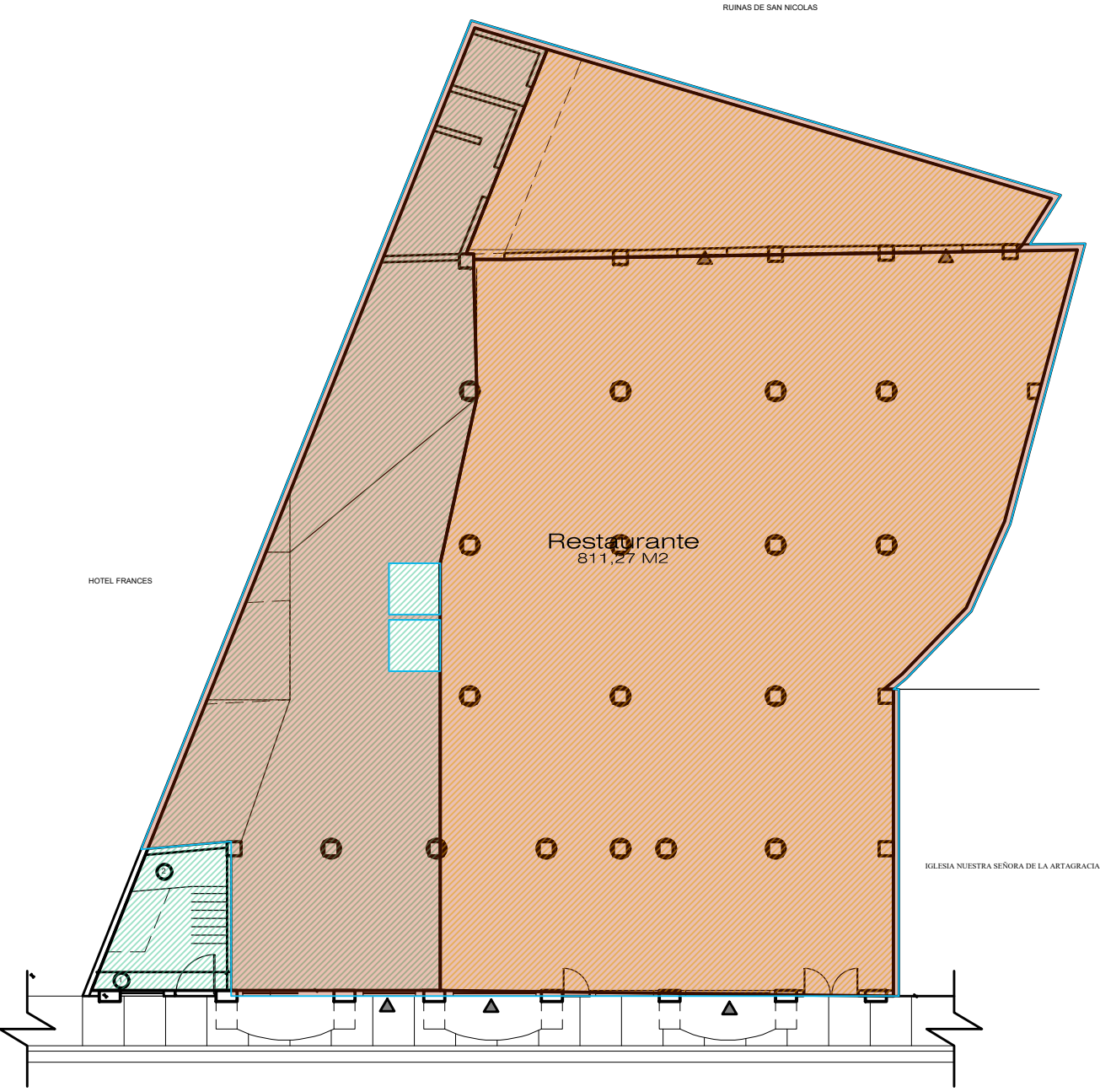
PLANTA PISO 1
